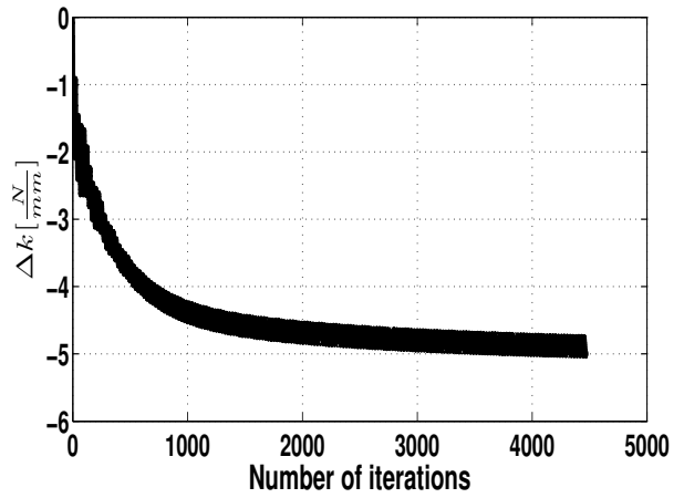
Fig. 5. Parameter k estimate
