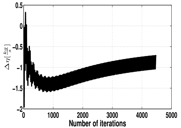
Fig. 6. Parameter \eta estimate
