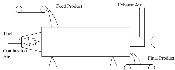
Fig. 1. Gypsum kiln
