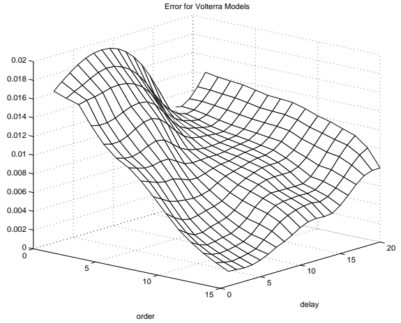
Fig. 5. Volterra Models
