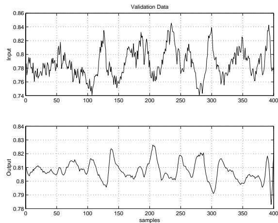
Fig. 8. Validation Data
